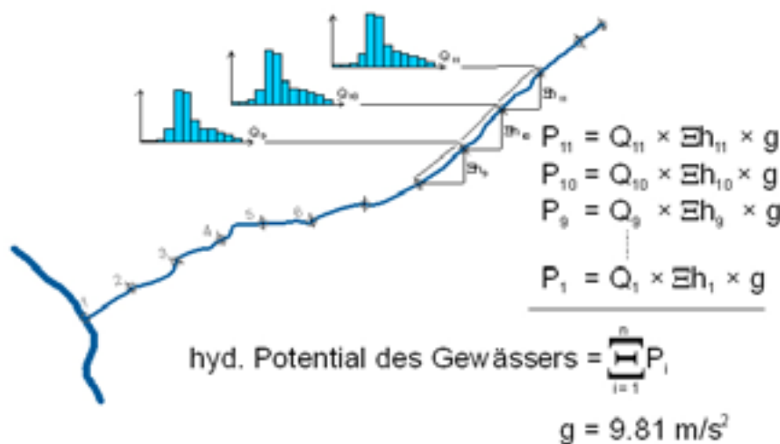
Figur 1: Ermittlung des Wasserkraftpotenzials für ein Gewässer (Prinzipskizze), basierend auf mittleren monatlichen Abflüssen für die Ermittlung des Kleinwasserkraftpotenzials der Schweiz (Quelle: Schröder 2009 [2])
