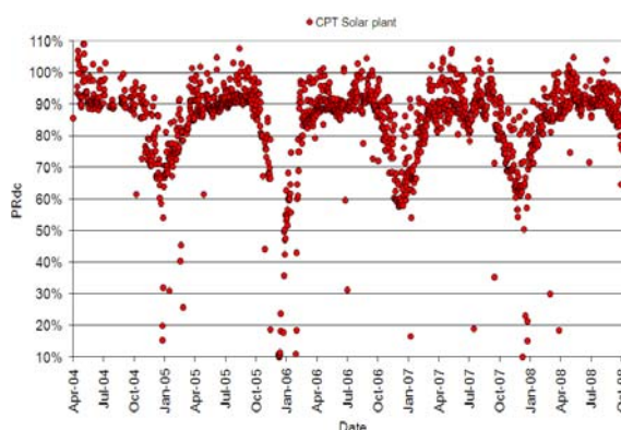
Figure 8: CPT Solar; modules solaires au silicium thermiquement isolés, depuis quatre années sans effets de dégradation (Source: ISAAC)
