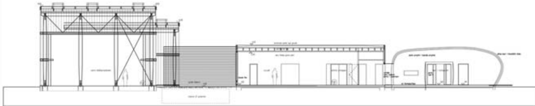
COUPE BB
