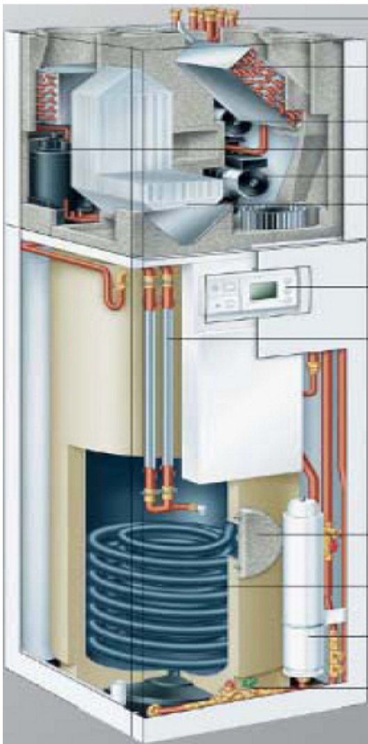
Figur 7: Kompaktgerät Viessmann/Vitotres 343
