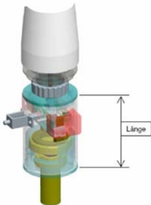
Figur 6: Optimierter Umkehrthermostatkopf (Miniaturisierung) (Bild: NTB/Schnyder)
